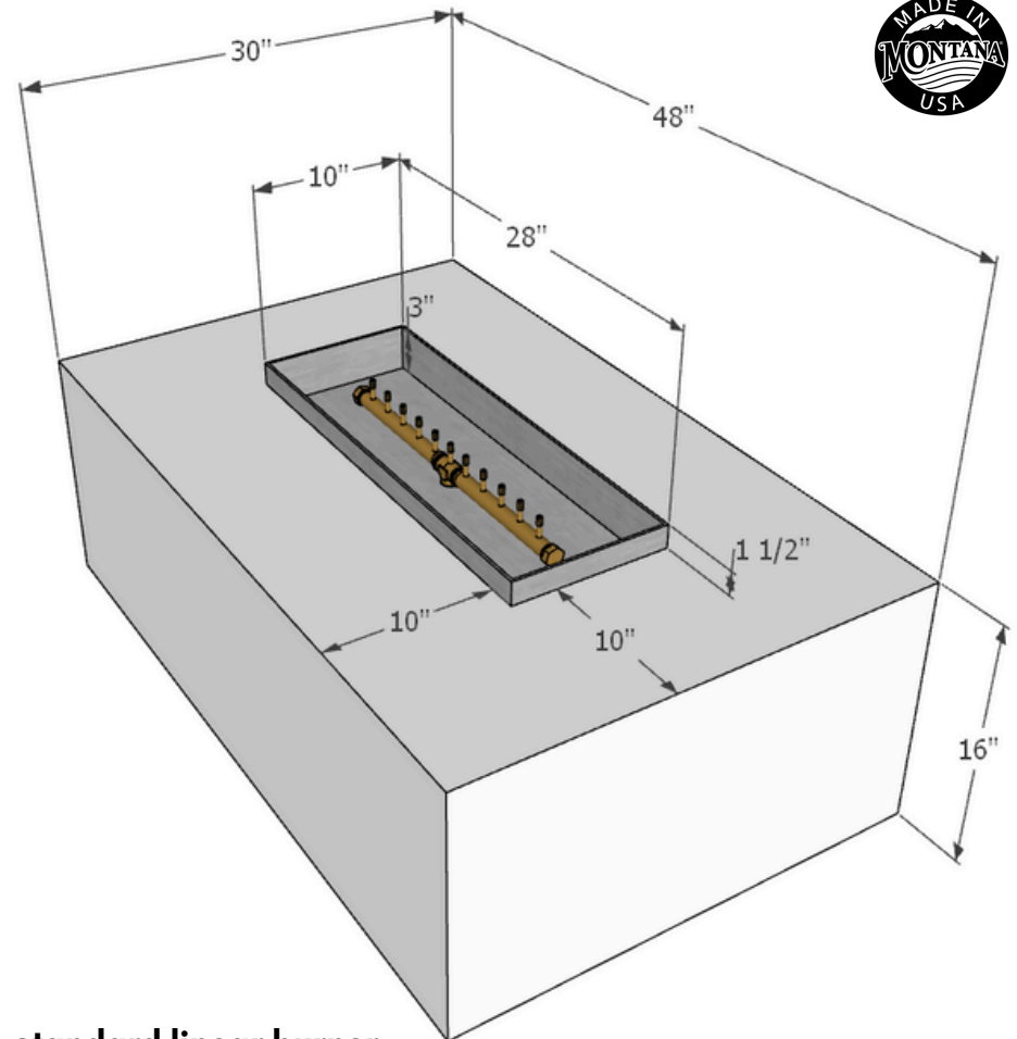
standard linear burner
