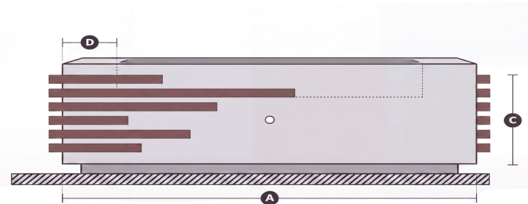
AAR.1 - 3 SIDE ELEVATION
